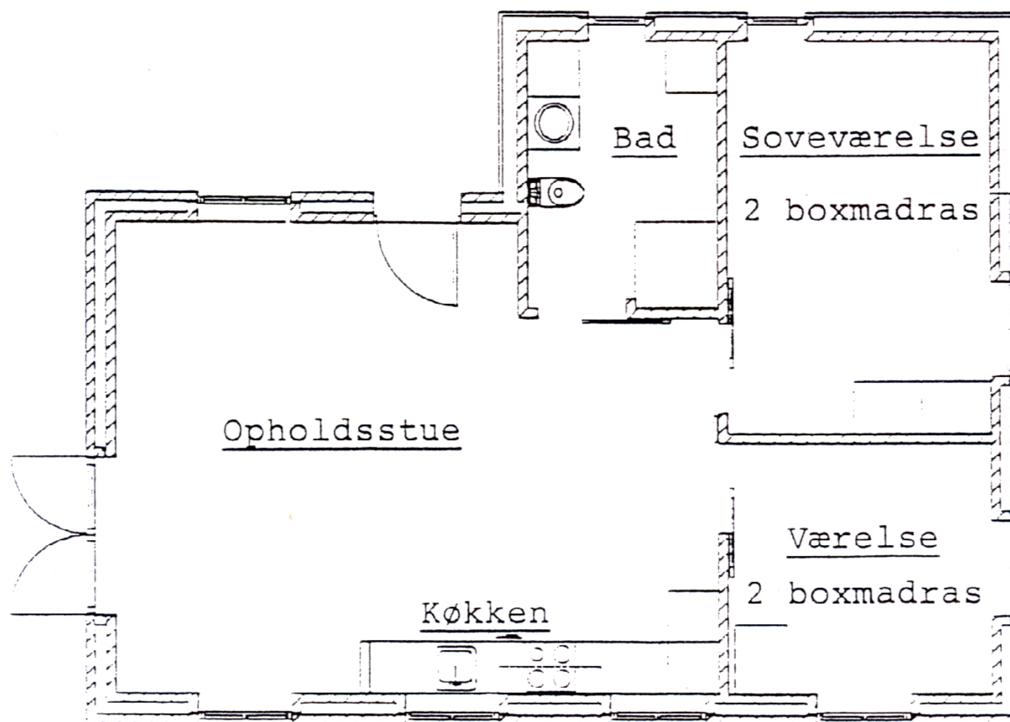
Stueetage
