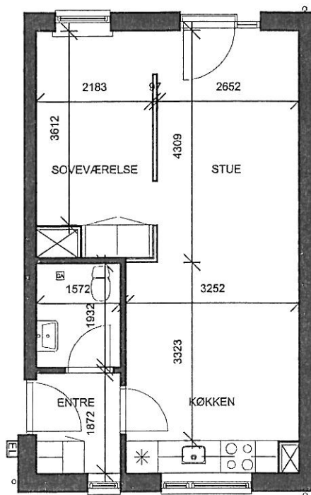
LEJLIGHED 3750, 1. SAL, 1:100 Alle mål er ca. mål og i mm.
