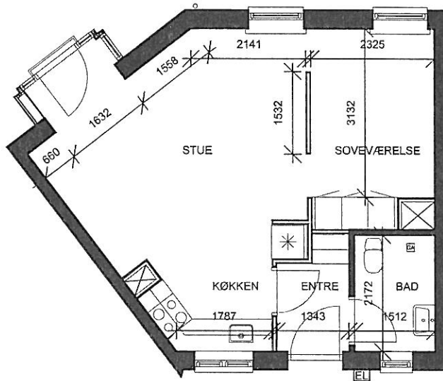
LEJLIGHED 3746, 1. SAL, 1:100 Alle mål er ca. mål og i mm.
