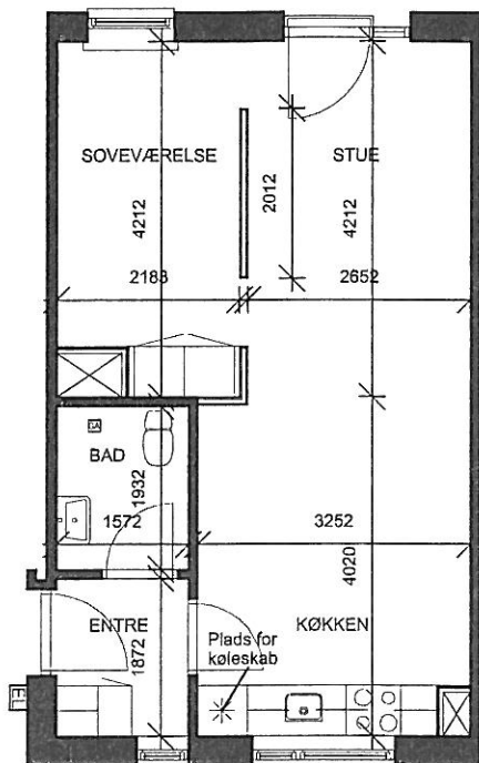
LEJLIGHED 3773, STUEETAGE, 1:100
