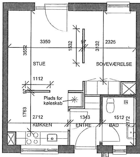
LEJLIGHED 3748, STUEETAGE, 1:100 Alle mål er ca. mål og i mm.
