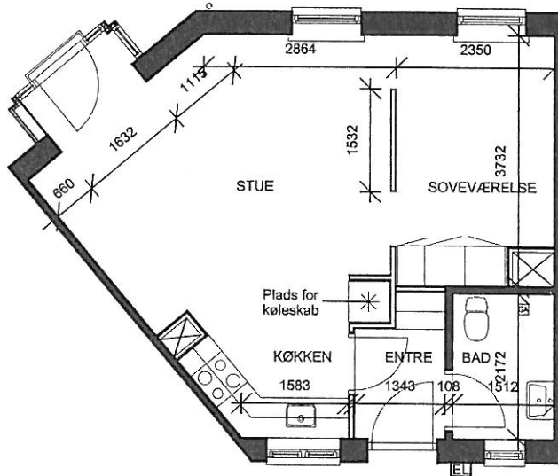
LEJLIGHED 3776, 1. SAL, 1:100 Alle mål er ca. mål og i mm.
