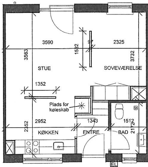
LEJLIGHED 3771, STUEETAGE, 1:100
